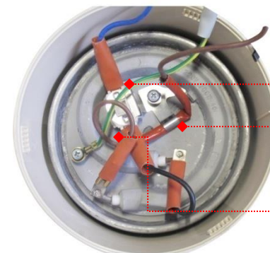
FSTB Thermostat
